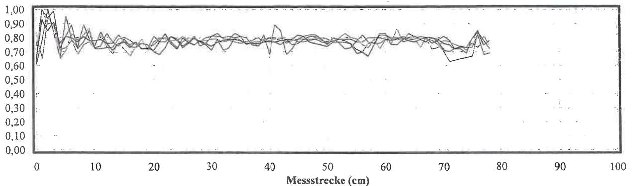
Gleitreibungskoeffizient [ \mu ]
