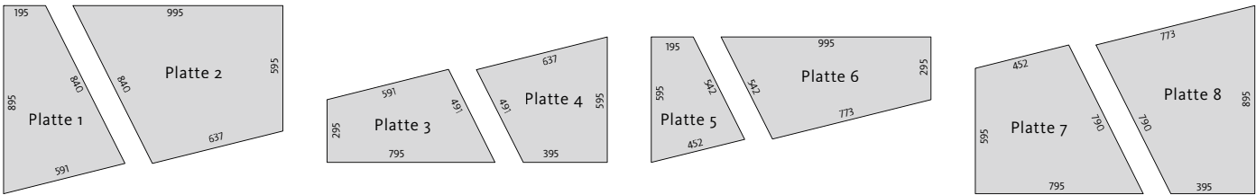
Platten 1–8 ergeben zwei Rauten
