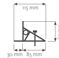
PAVE-EDGE STARRFLEX Befestigungsschiene kurvige Begrenzungen (befahrbar) Baulänge 240 cm
