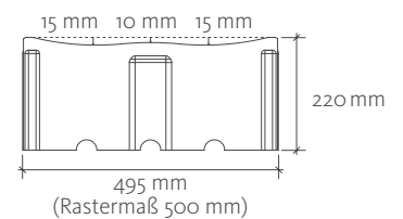
Rinnenstein
