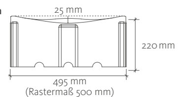
Übergangstein
